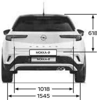
המידות במ"מ
